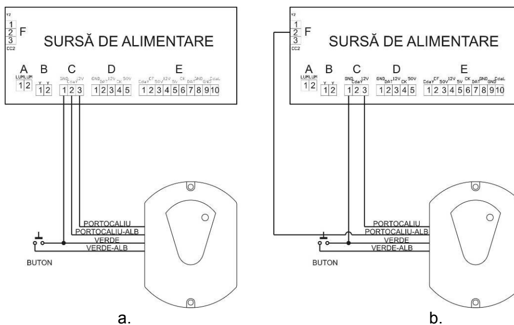
Fig. 1 Conectare cititor de proximitate la sursă de alimentare tip SA-ISCP
