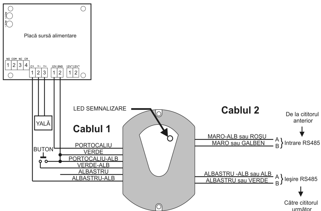
Fig. 1 Schiță conectare cititor PROXA 01 MF RS485 și Yală electromagnetă la sursa SA SIMPLA
