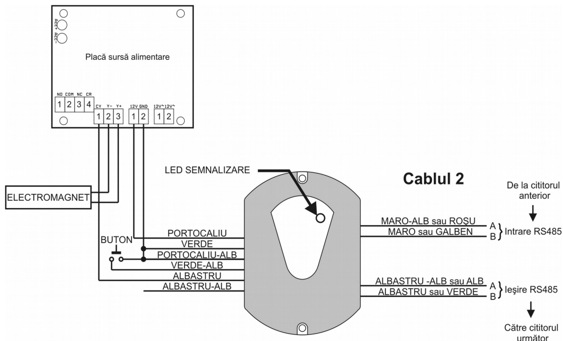
Fig. 2 Schiță conectare cititor PROXA 01 MF RS485 și Electromagnet la sursa SA SIMPLA
