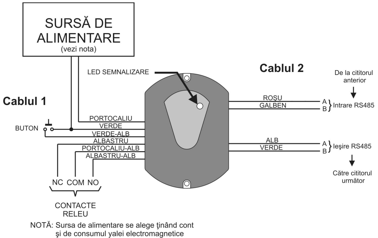
Fig. 1 Schiță conectare cititor PROXA 01 MF RS485
